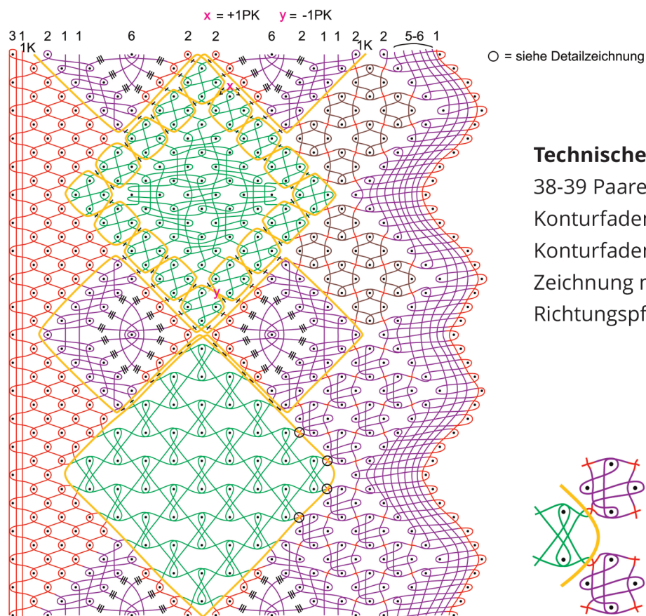
Abb. 57a: Technische Zeichnung.
